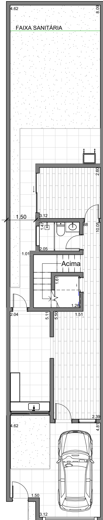
LEGAL-001-Terreo 1 : 100
